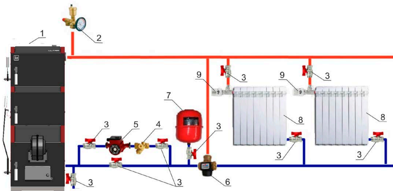
Рис. 5 Схема подключения котла к закрытой системе с принудительной циркуляцией теплоносителя с термостатическим смесительным клапаном
