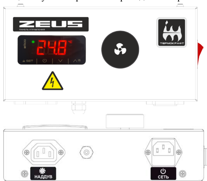
Рис. 7 Панель управления котла ULTRA
