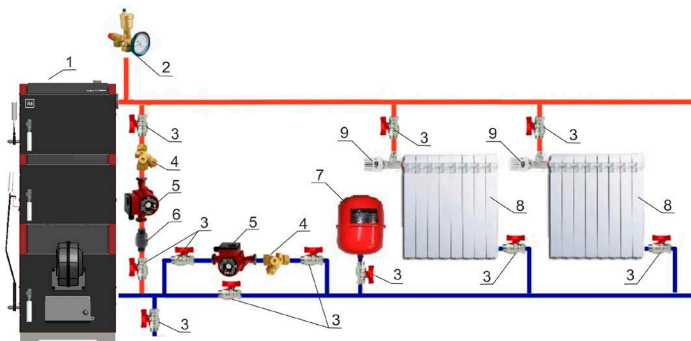
Рис. 4 Схема подключения котла к закрытой системе с принудительной циркуляцией теплоносителя с рециркуляционным насосом
