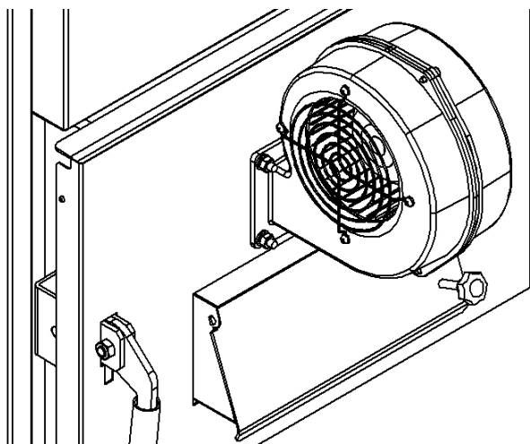
Рис. 6 Установка вентилятора наддува
