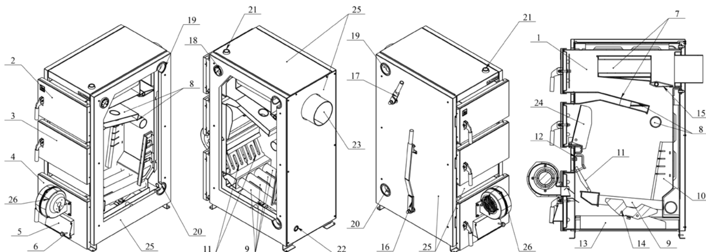
Рис. 1 Устройство котла
